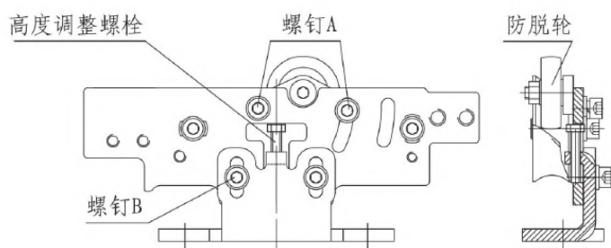
吊架组件(二)
