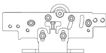
吊架组件(一)
