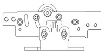
吊架组件(二)
