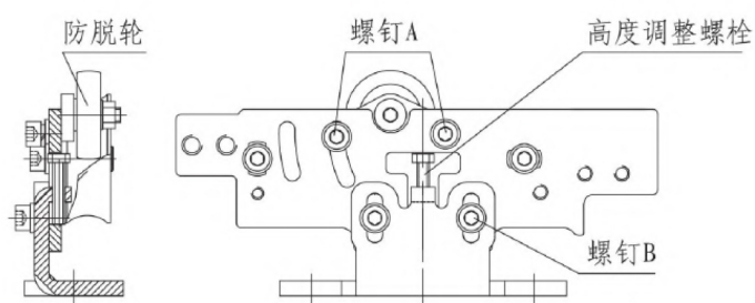
吊架组件(二)
