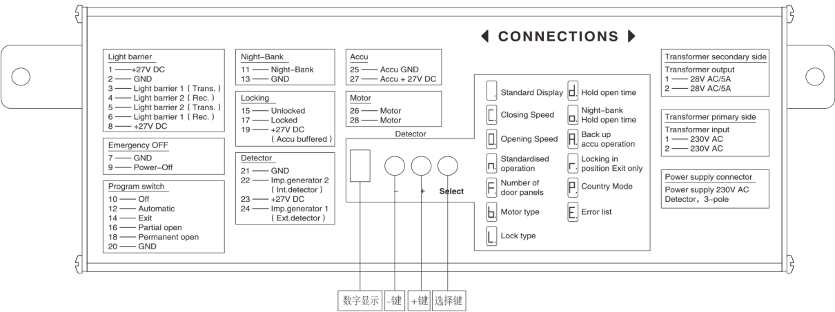
控制器左端
