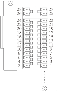
控制器左端
