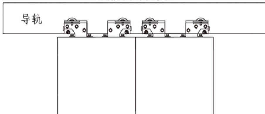
双扇门吊架安装图
