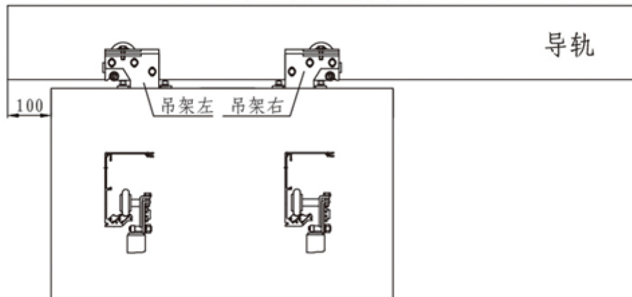
单扇右开吊架安装图
