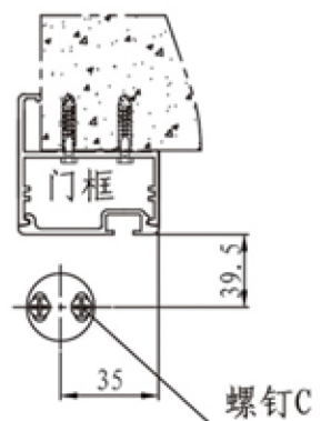
左开门地轮安装示意图
