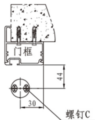
右开门地轮安装示意图
