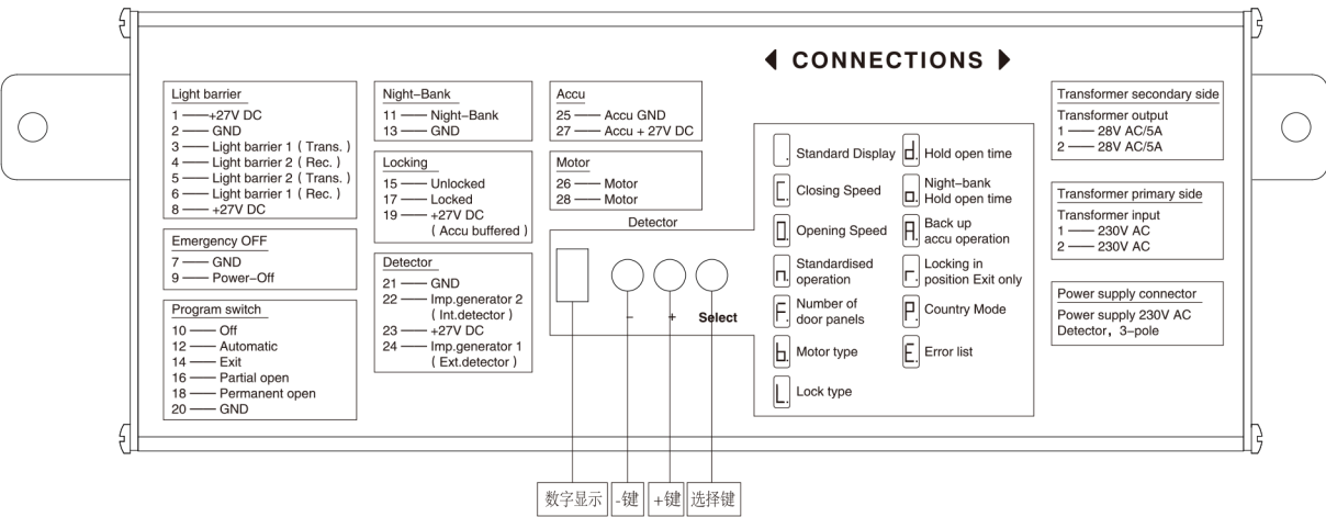
控制器左端
