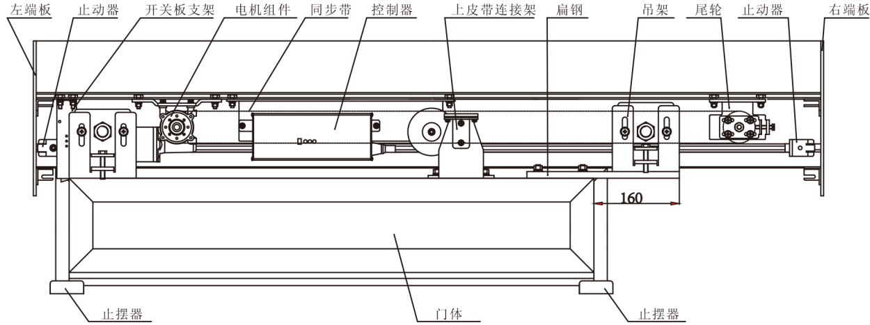
单扇右开型
