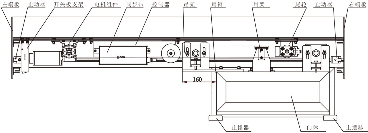
单扇左开型
