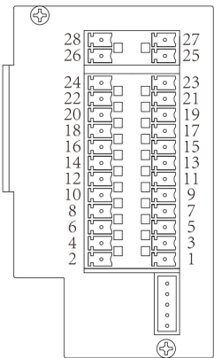
控制器左端
