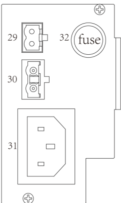
控制器右端
