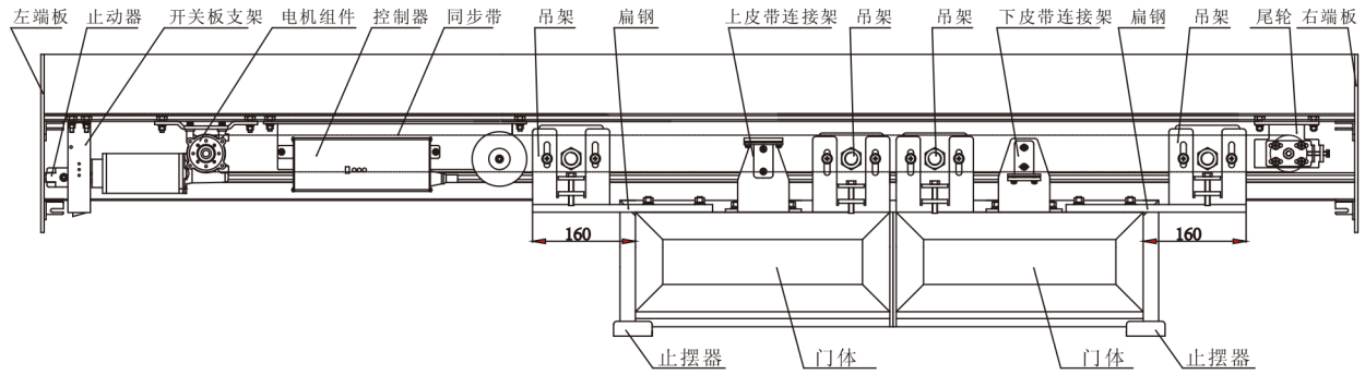
双扇对开型
