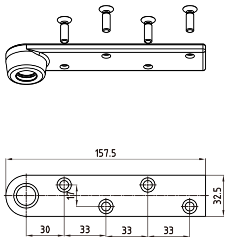
支架下附件
