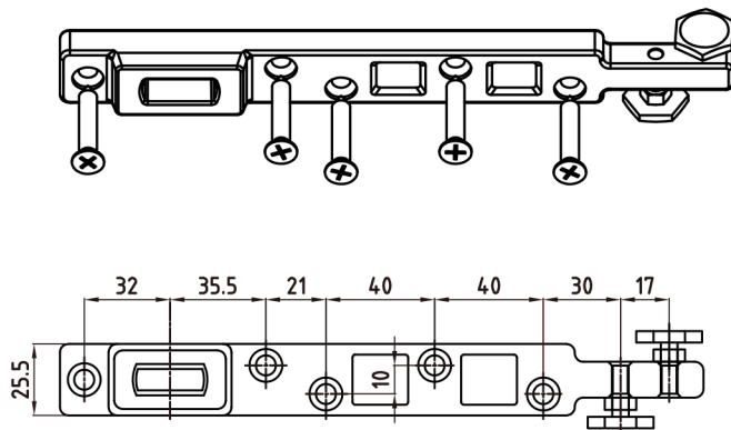
转动臂杆组件
