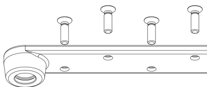
支架下附件
