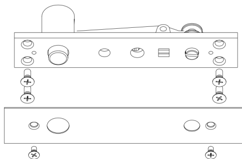
支架上附件
